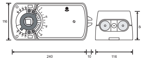
尺寸 (mm)
