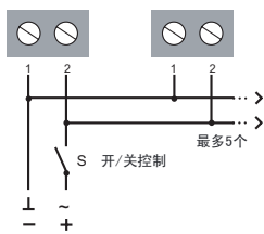
接线图
