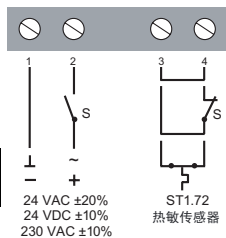
控制接线图
